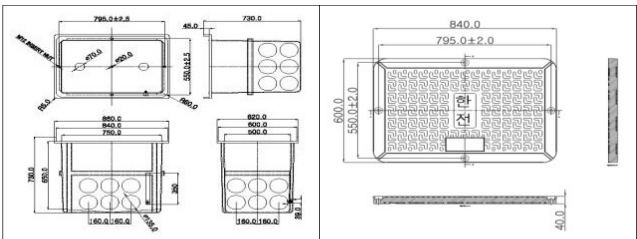
[그림 1] 배전용 FRP 저압 접속함체 및 뚜껑
